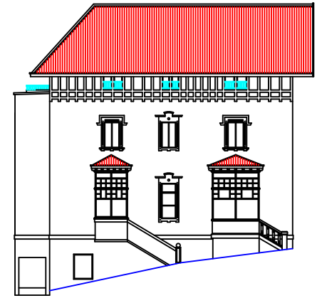
Ezkerreko fatxada
