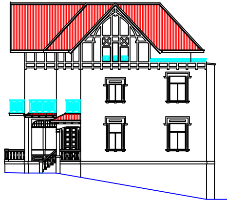
Eskuineko albo-fatxada
